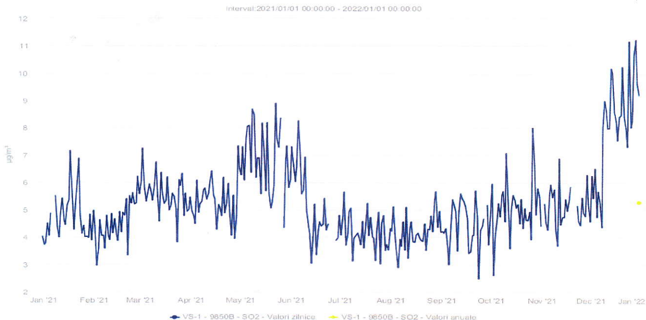
Fig. 2.4. Concentrații medii zilnice pentru indicatorul SO 2 , măsurate la stația VS-1, anul 2021
